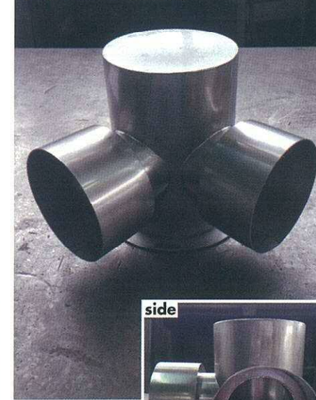
ステンレス 製罐品
